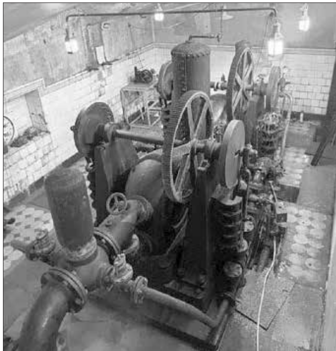
Blick auf das vollständig erhaltene Peltonrad-Pumpwerk im historischen Wasserwerk Vielbrunn. Die Anlage ist am Rahmen des Tags des offenen Denkmals am 8. September für die Öffentlichkeit zugänglich.
